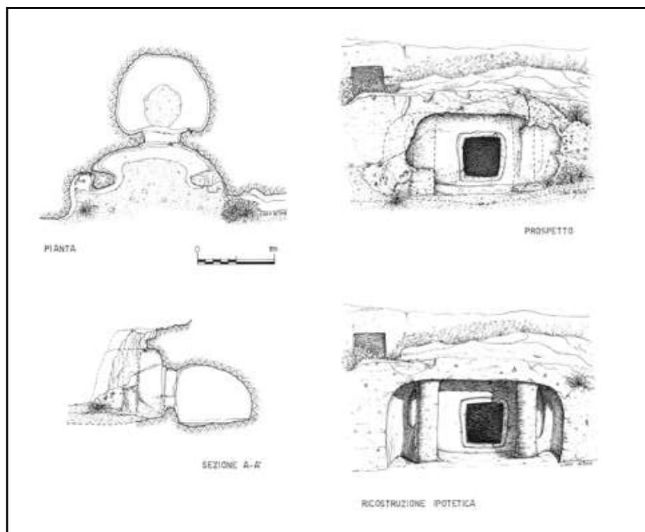
Fig. 2 - Necropoli di Predio Reale (SR). Tomba 1: pianta, sezione, prospetto e ipotesi ricostruttiva del prospetto (dis. G. Libra).
