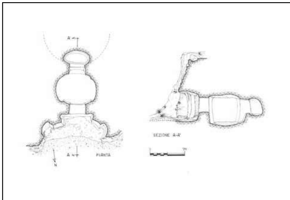
Fig. 4 - Necropoli di Predio Reale (SR). Tomba 10: pianta e sezione (dis. G. Libra).
